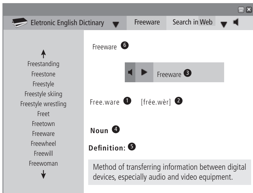
Figura 3.2: Dicionário Eletrônico
