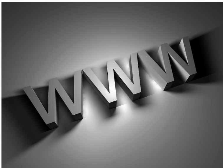
Figura 1.2: WWW
