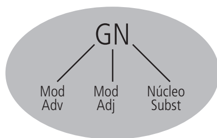
Figura 4.1: Grupos nominais
